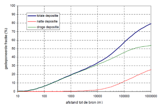
Figuur 1b: Fractie van gedeponeerde \text{NH}_3 als functie van de afstand tot de bron, gemiddeld over alle windrichtingen met een bronhoogte van 3 m (uit Kros, et. al., 2008)
